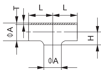
Pull tee L7WWW
