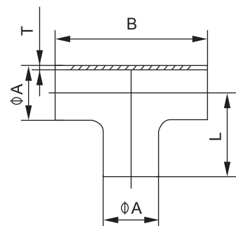
Equl tee
