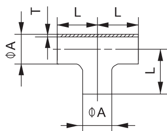
Equal tee D.7W
